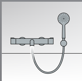
Wannenthermostat mit integriertem Wanneneinlauf und Umsteller zu Handbrause
